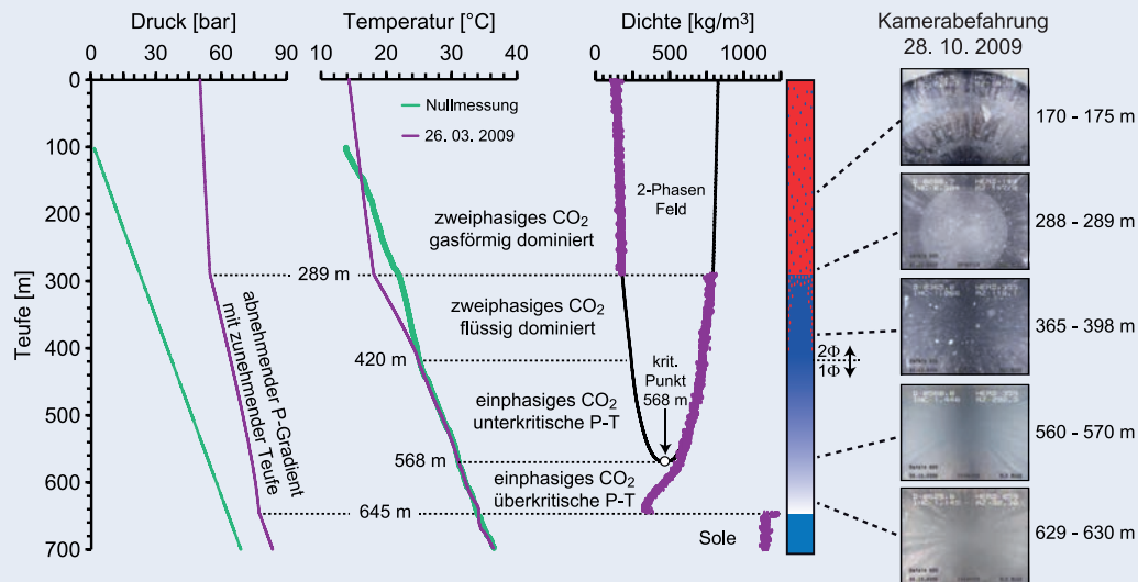
Abb. 5: P-T-Profil der Bohrung Ktzi 200 für die Nullmessung vor Beginn der Injektion sowie eine Loggingkampagne im März 2009 (links), die aus den Daten der Loggingkampagne abgeleiteten Phasenzustände in der Bohrung (Mitte) sowie Ergebnisse der Kamerabefahrung der Ktzi 200 (rechts)
